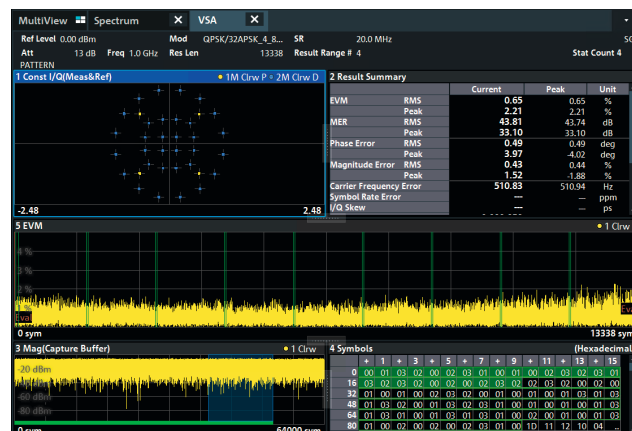
Демодуляция сигнала DVB-S2X с несколькими модуляциями с помощью опции R&S®FPL1-K70M (требуется опция R&S®FPL1-K70)
